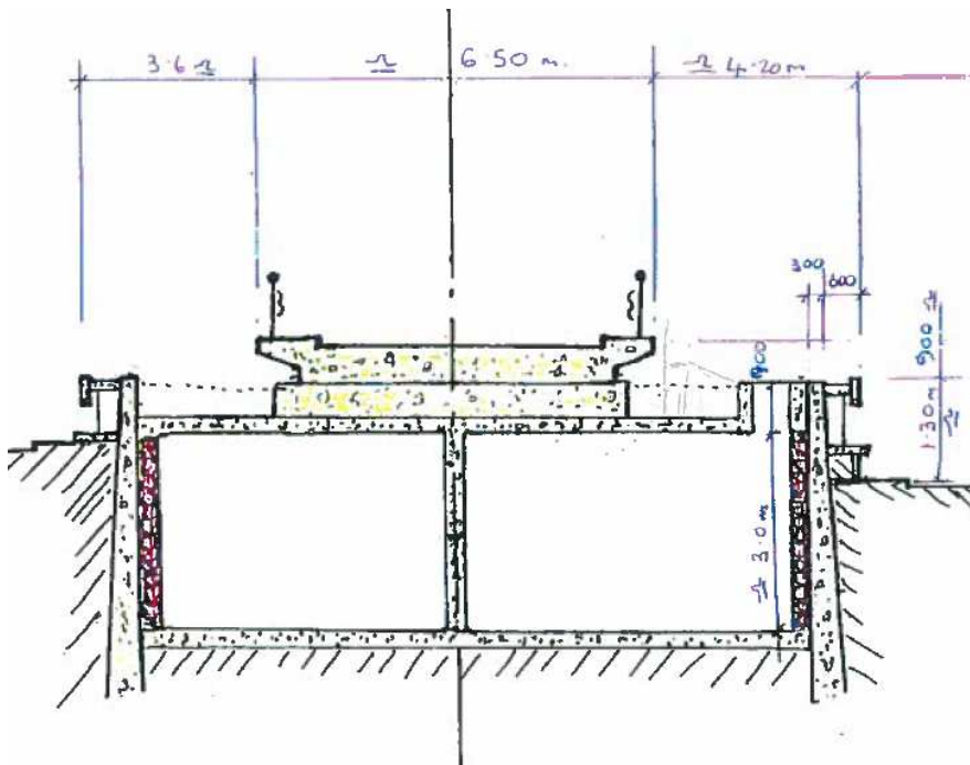
Τυπική Τομή Οχετού
