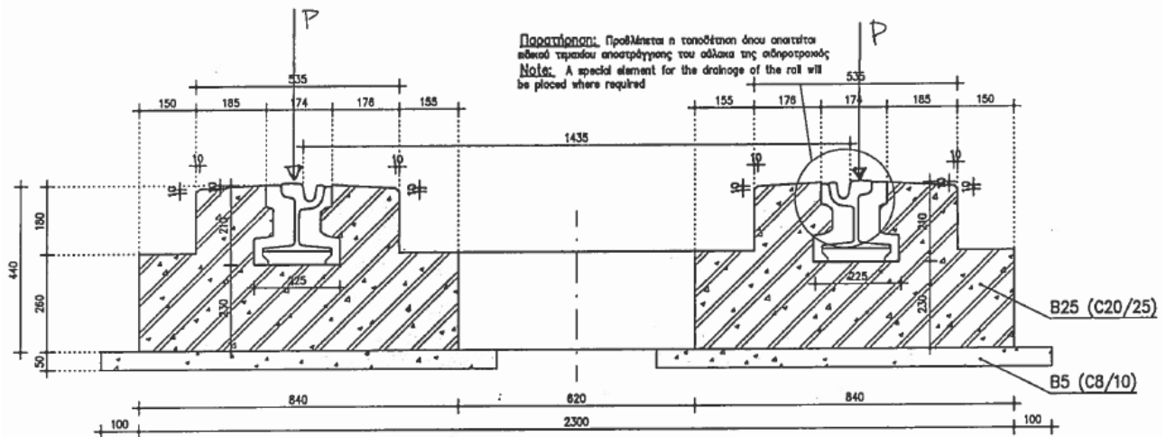
ΤΥΠΙΚΗ ΤΟΜΗ / TYPICAL SECTION Κλ. 1:10 / SC. 1:10
